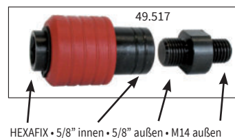
49.517 HEXAFIX • 5/8" innen • 5/8" außen • M14 außen Somit kann nahezu jedes Rührwerk mit einer HEXAFIX-Schnellkupplung nachgerüstet werden.
